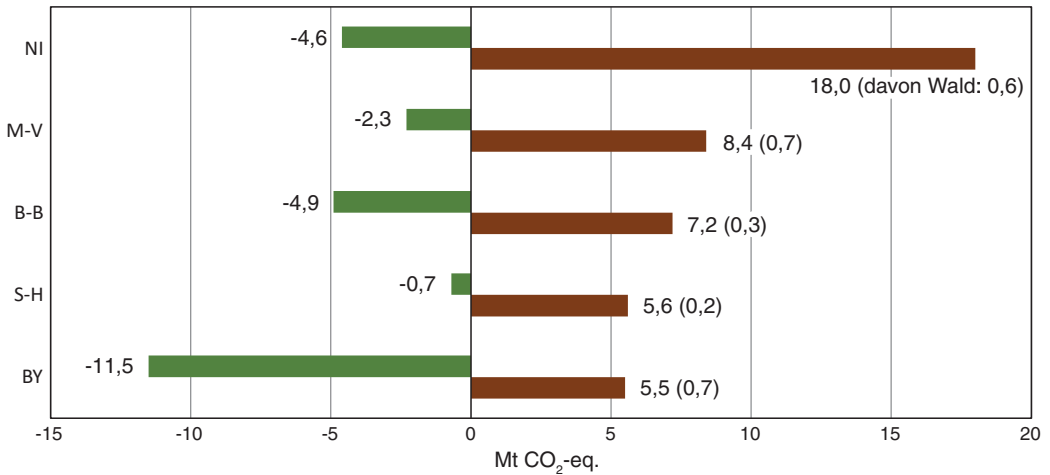
Abb. 7. Treibhausgasemissionen aus organischen Böden (■, Emission aus Moorwaldflächen in Klammern) der fünf moorreichen Bundesländer im Vergleich zur Kohlenstoffbindung in Wäldern (■, Senkenfunktion) im Jahr 2020; NI: Niedersachsen, M-V: Mecklenburg-Vorpommern, B-B: Berlin-Brandenburg, S-H: Schleswig-Holstein, BY: Bayern. – Greifswald Moor Centrum (2023).
