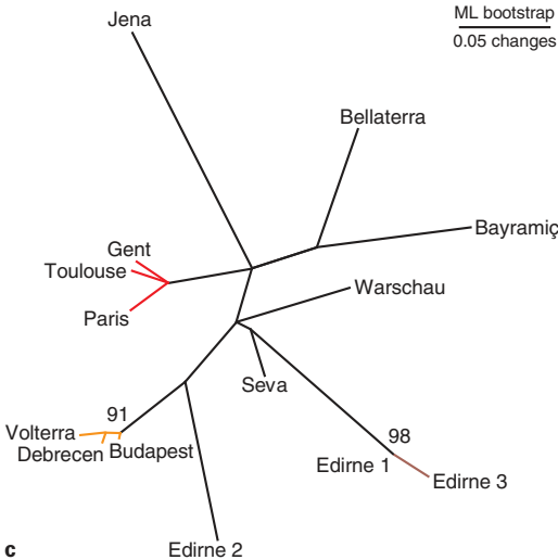
Abb. 8. Lasius neglectus : a, Standorte der 14 untersuchten eingeführten Populationen; b, über Aggressionstests erstellte Cluster der 14 Populationen; c, phylogenetischer Stammbaum der kooperativen Cluster (6 Mikrosatelliten-Loci). – © Ugelvig et al. (2008), CC-BY-2.0.
