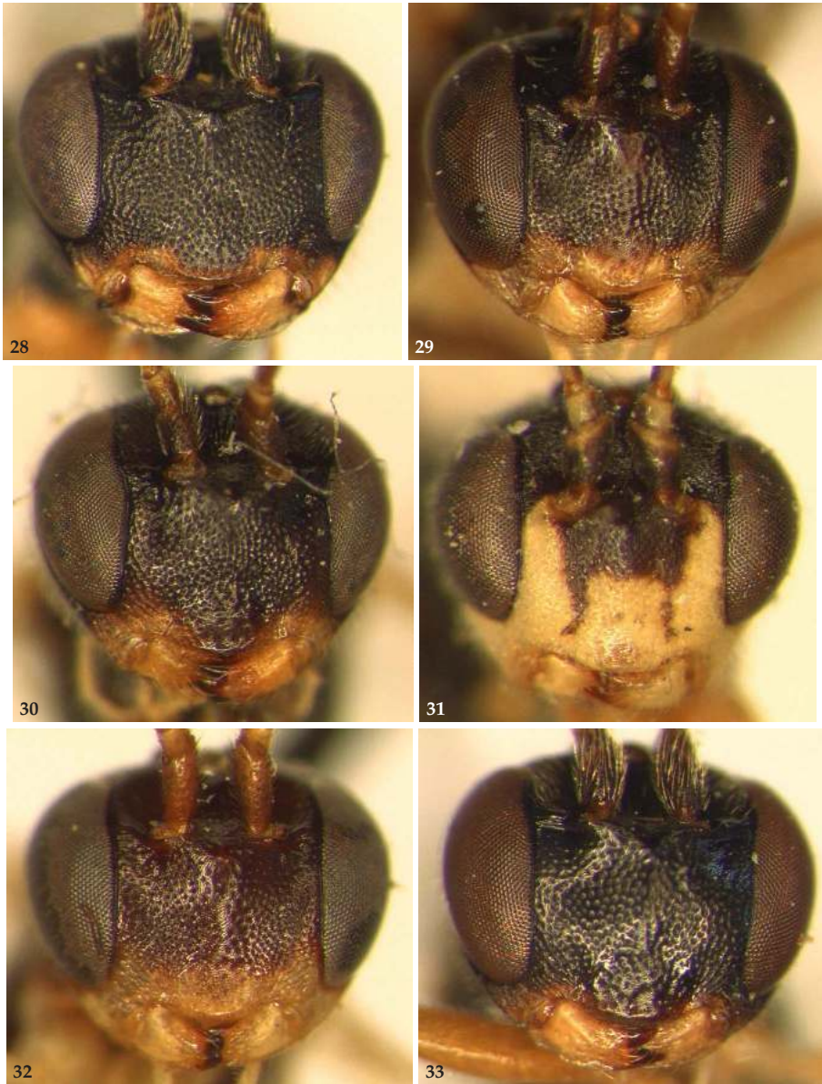
Figs 28–33. Face of ♀♀ from frontal: 28. A. diversum Schwenke; 29. A. dorsale (Holmgren); 30. A. flagellator spec. nov.; 31. A. flavoventrale spec. nov.; 32. A. hirsutum (Bridgman); 33. A. italicum Schwenke.
