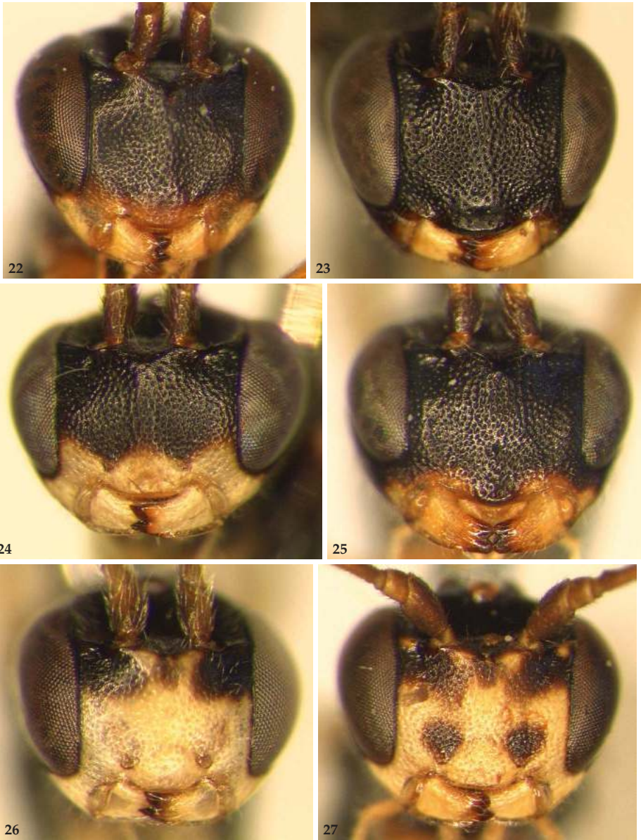
Figs 22–27. Face of ♀♀ from frontal: 22. A. aggressor (Fabricius); 23. A. albitarse (Brischke); 24. A. alpinum Roman; 25. A. buccatum (Thomson); 26–27. A. anale (Holmgren).
